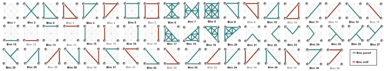
Fig. 1. Bibliothèque de blocs flexibles passifs et actifs implémentés dans FlexIn.
