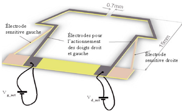
Fig. 6. Vue CAO de la micropinçe piézoélectrique mettant en évidence les zones dédiées à l'actionnement et la mesure.
