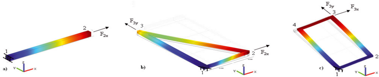
Fig. 5. (a) Bloc piézoélectrique 13 et sa déformée, où le nœud 1 est bloqué, ( L_{12} = 3 mm, h_{12} = 150 \mu m, e_p = 200 \mu m); (b) bloc piézoélectrique 3 et sa déformée, où le nœud 1 est bloqué, ( L_{12} = 3 mm, h_{12} = 150 \mu m, L_{13} = 6 mm, h_{13} = 300 \mu m, L_{23} = 6.708 mm, h_{23} = 167.7 \mu m, e_p = 200 \mu m); (c) bloc piézoélectrique 5 et sa déformée, où le nœud 1 est bloqué, ( L_{12} = 3 mm, h_{12} = 150 \mu m, L_{13} = 6 mm, h_{13} = 300 \mu m, e_p = 200 \mu m).
